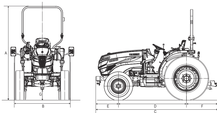
TG6407 MET VEILIGHEIDSBEGEL ACHTERAAN
