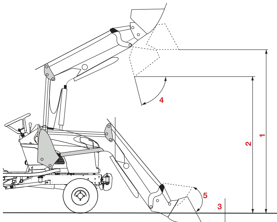
4-IN-1 BAK Beschikbaar op frontlader met werktuigdrager
